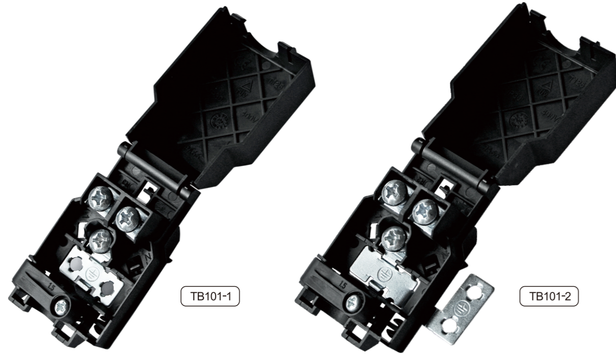
接线盒2/3
